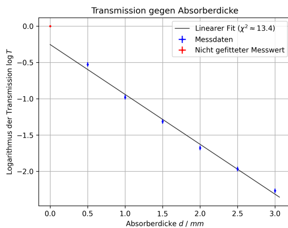
Abbildung 22: Linearer Fit des Logarithmus des Transmissionsgrads \log T gegen Absorberdicke d (Molybdän-Röhre, U = 35 \text{ kV} , ohne Zirkoniumfilter)
