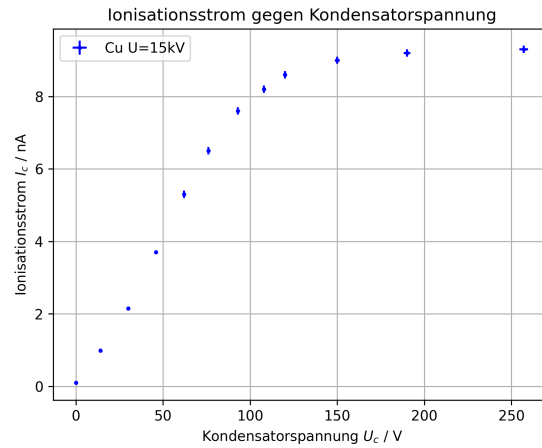
Abbildung 10: Ionisationsstrom I_C des Kondensators in Abhängigkeit der Kondensatorspannung U_C für Röhrenspannung U = 15 kV (Kupfer-Röhre, I = 1 mA)
